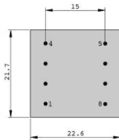
Ansicht auf die Stifte
